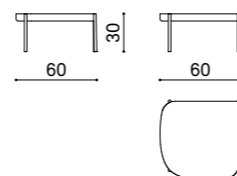
AB TCS0 coffee table tavolino table basse
