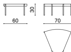
AB TCX0 coffee table tavolino table basse
