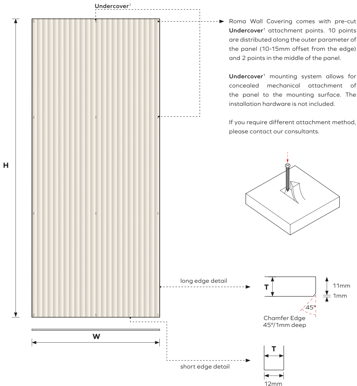
Dimensions table 2
