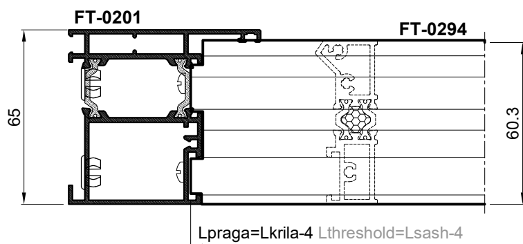
MJERA PILANJA PRAGA CUTTING LENGTH
