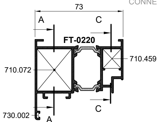
PRESJEK B-B CROS-SECTION B-B
