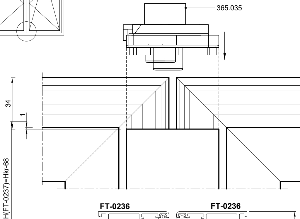
365.035 - UMETAK ZA PROFIL FT-0237- ZA KRILO PROZORA (pvc) 365.035 - INSERT FOR PROFILE FT-0237 - FOR WINDOW SASH (pvc)
