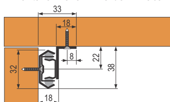
Montaža mehanizma bez krilaca
