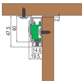
Prikaz montaže mehanizma
