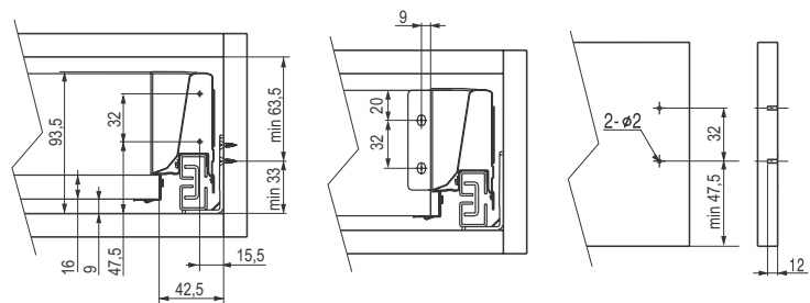
Dimenzije za montažu niske fioke
