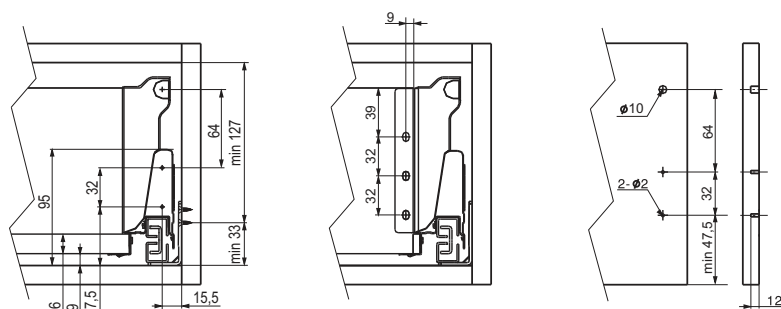
Dimenzije za montažu visoke fioke
