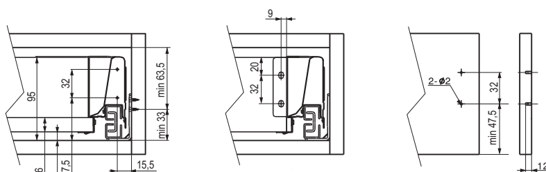
Dimenzije za montažu niske fioke
