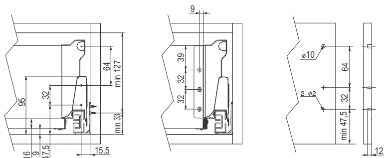
Dimenzije za montažu visoke fioke
