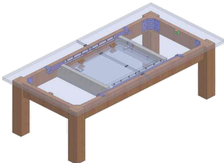
2. Prikaz otvorenog HMR mehanizma
