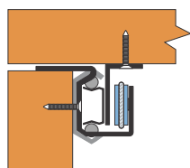
Montaža mehanizma sa krilcima
