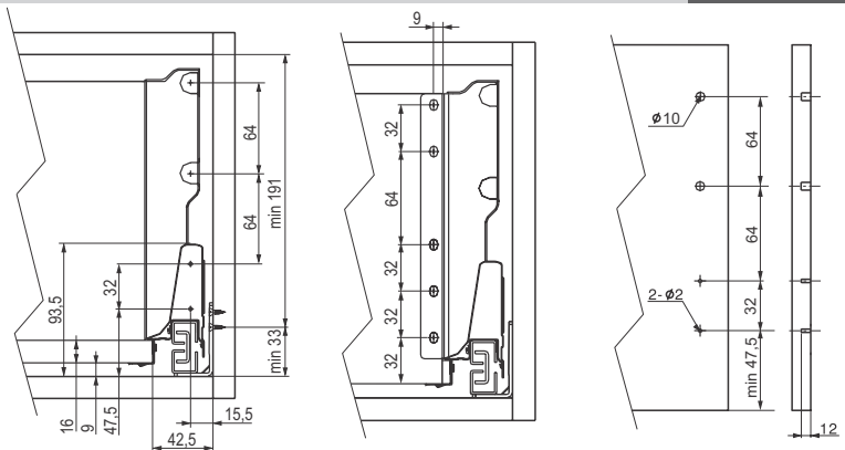
Dimenzije za montažu visoke fioke
