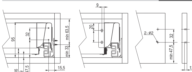
Dimenzije za montažu srednje fioke
