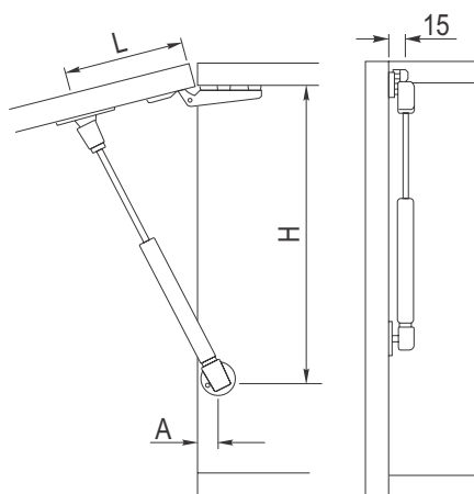
Prikaz montaže standardnog amortizera
