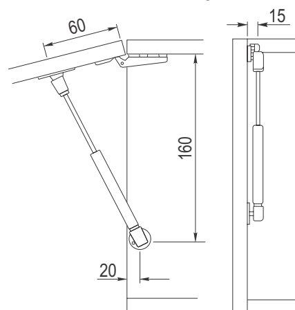
Prikaz montaže kratkog amortizera
