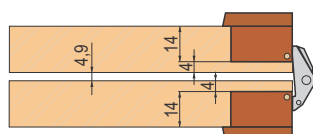
Pozicioniranje šarke za umetak
