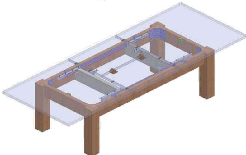
3. Prikaz rasklopljenog mehanizma sa umetkom
