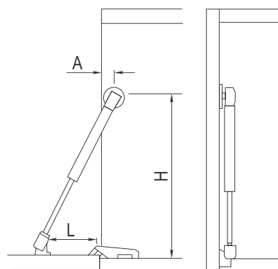
Prikaz montaže bife amortizera
