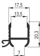
TAB 4837 Al donji ram profil
