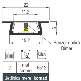
LED senzor dodira / 2m UGRADNI
