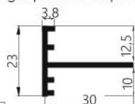
Al. ger profil za stepenište
