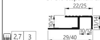
ST 310 stepenišni al. profil
