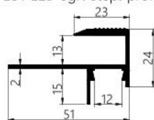
Protivklizni profil
