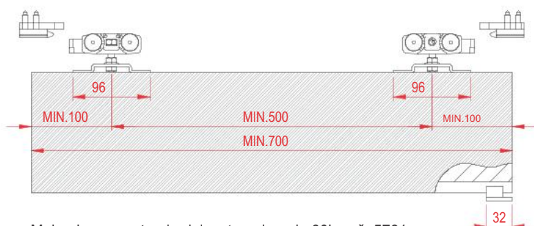
Mehanizam sa standardnim stoperima do 60kg - š: 5761
