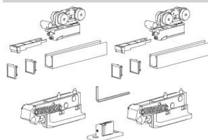
PVD TS-EVOLUTION/80 meh.-usp.
