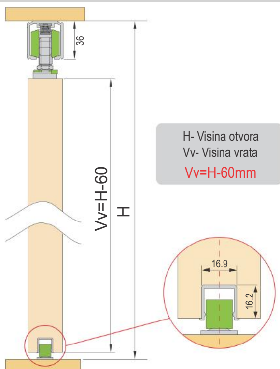
PVD CFB gornja 1k šina AL (PVS)
