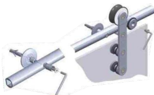
Prikaz montaže stopera i montiranja šine na zid
