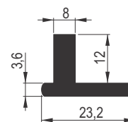
Usmerivač pravca PVC
