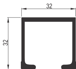
PVD SKS 51 gornja 1k šina
