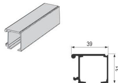
PVD TS-1700 gornja šina AL (PVS)
