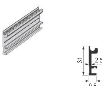
PVD TS-1700 nosač 1720 AL (PVS)
