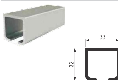
PVS EP-03 al.gornja šina
