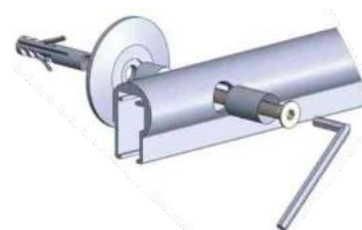
Prikaz montaže tiplova i distancera za gornju šinu
