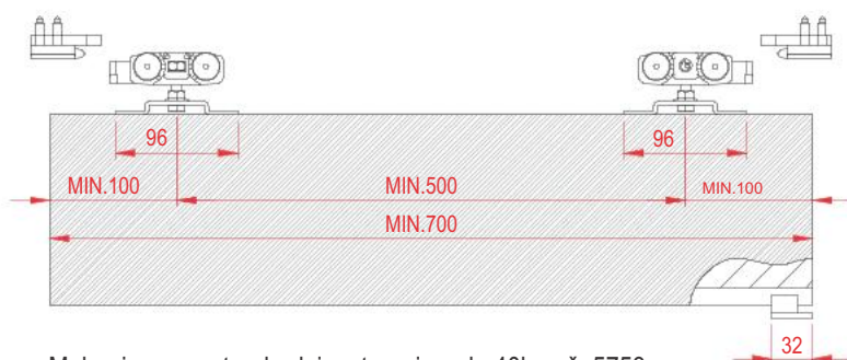
Mehanizam sa standardnim stoperima do 40kg - š: 5753
