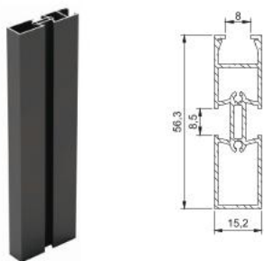
UPGS vertikalni profil AL
